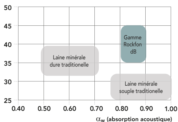
D_{n,f,w} (isolation acoustique)
