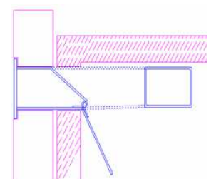
Coffre TA 1212 Tiroir Pour Mur Epaisseur 350 mm
