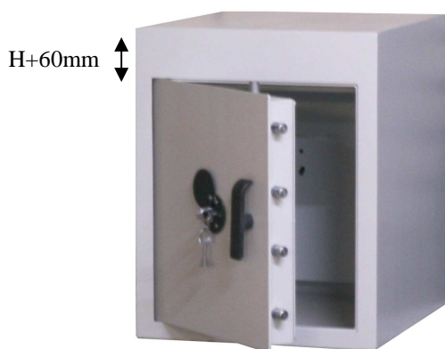
TA 84 B5 avec ASERVISSEMENT MECANIQUE DES portes Façade 8 ou 12 mm Caisse 4mm
